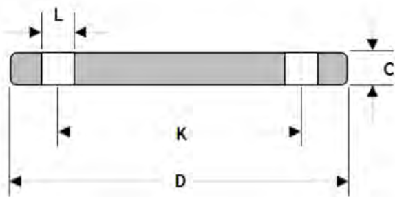
PN16 F/F BLANK FLANGE 316 - E THICK
